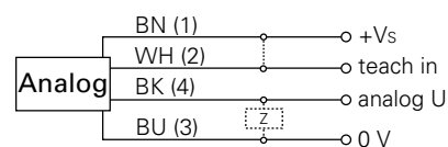
连接图
