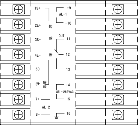
电气连接图
